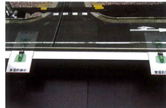
サーモクロンGで、30分間隔温度測定装置セット
